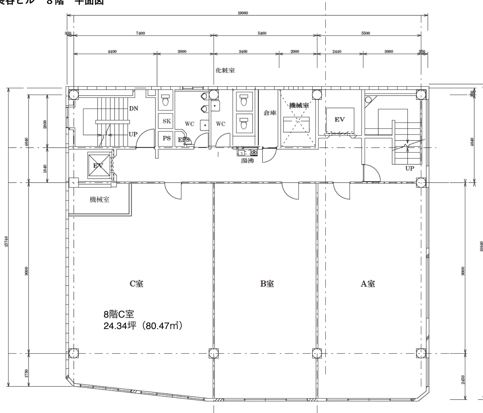
六角長谷ビル 8階 平面図
