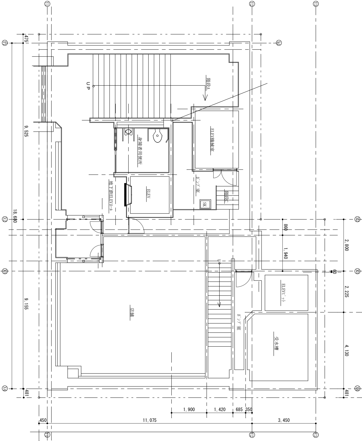
四ツ橋長谷ビル4階平面図1/100
