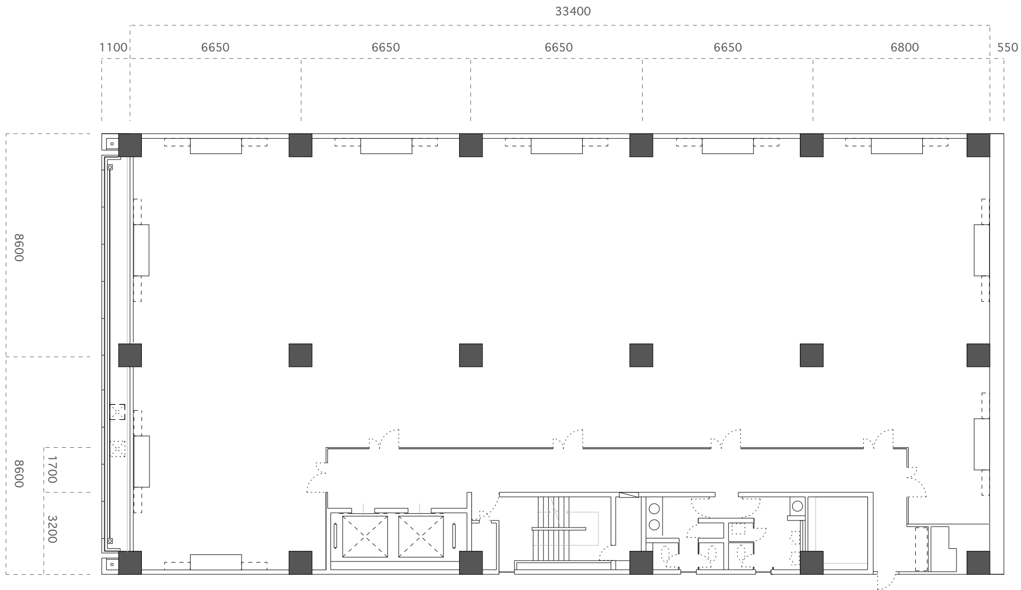
第八長谷ビル 平面図
