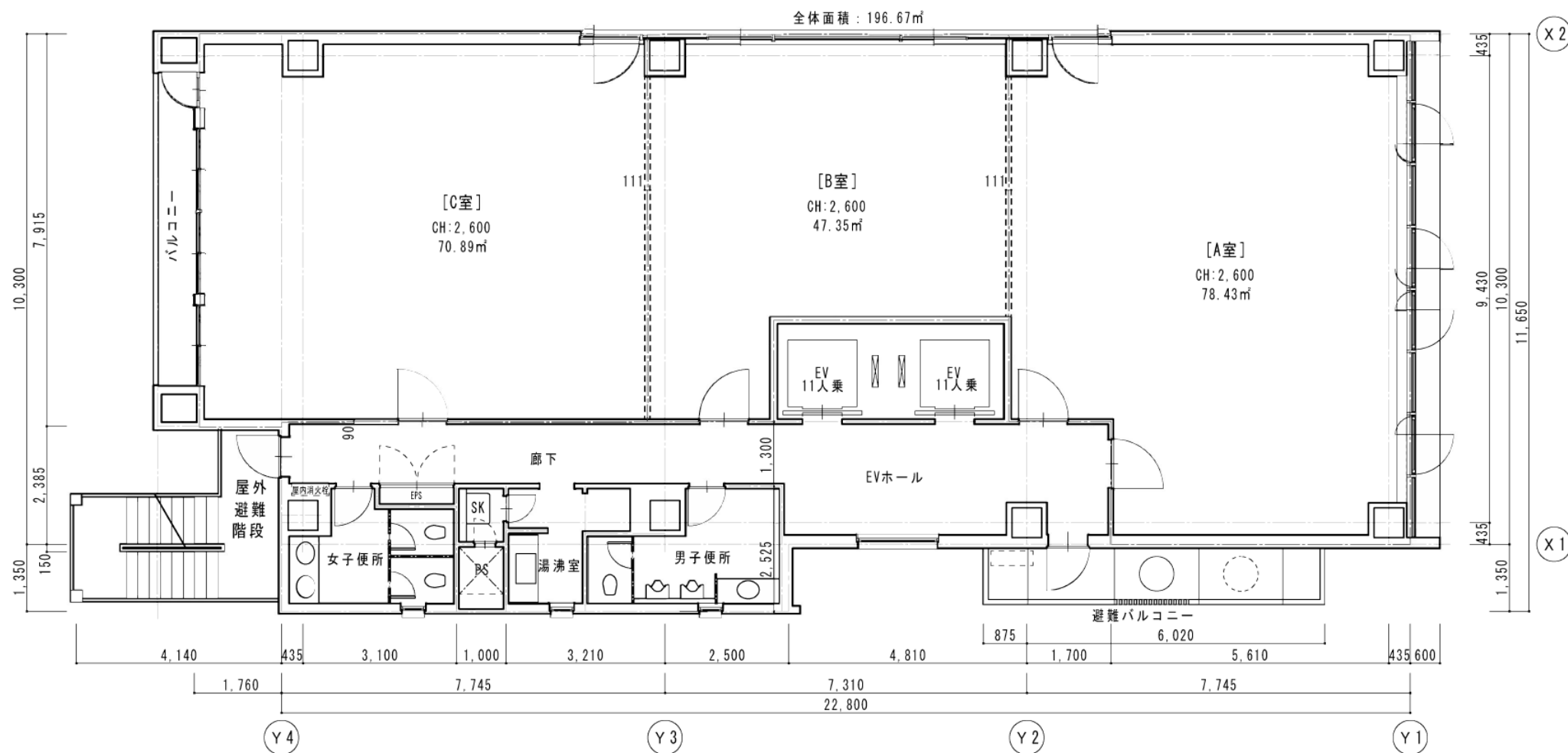
第 14 長谷ビル 基準階平面図
