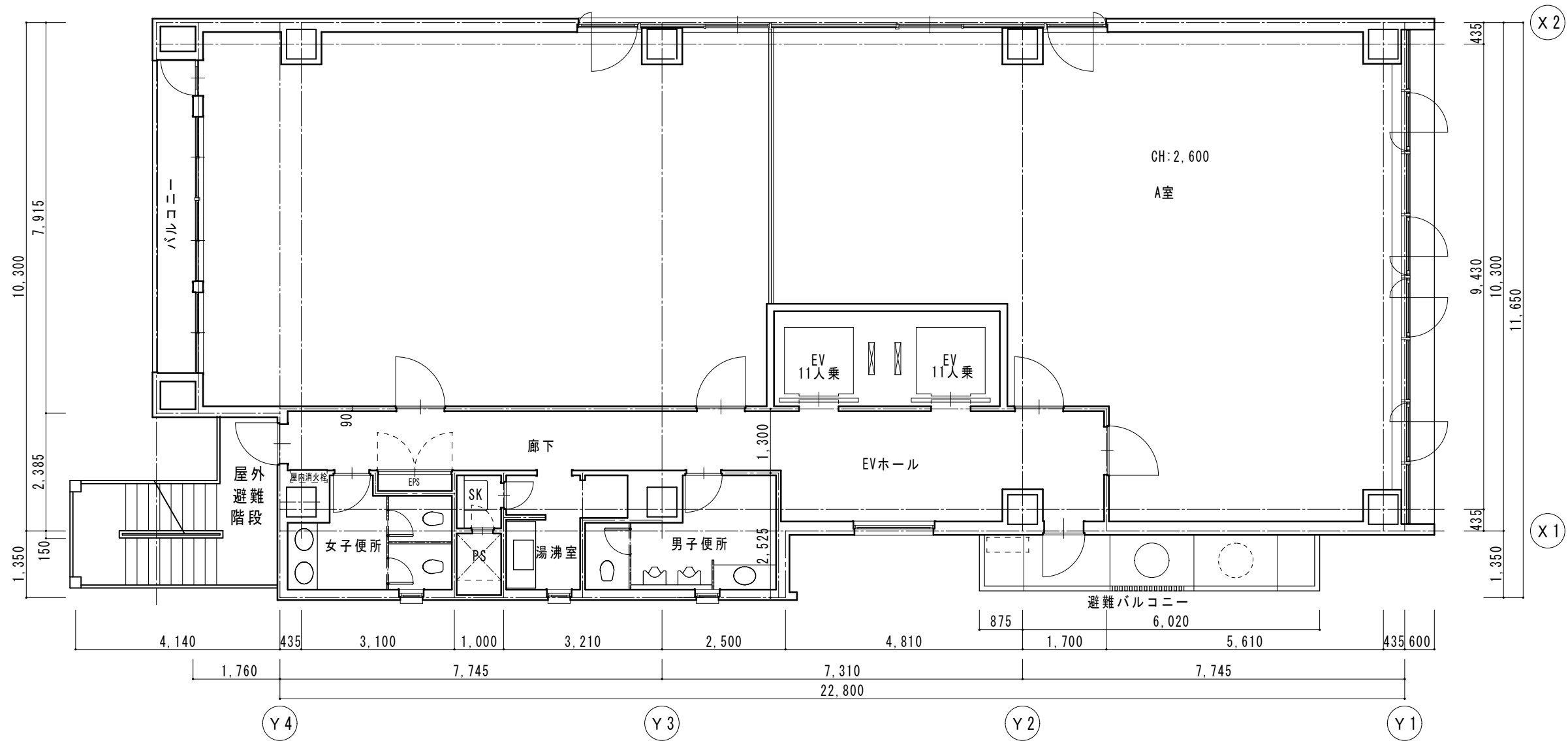
【9階平面図】
